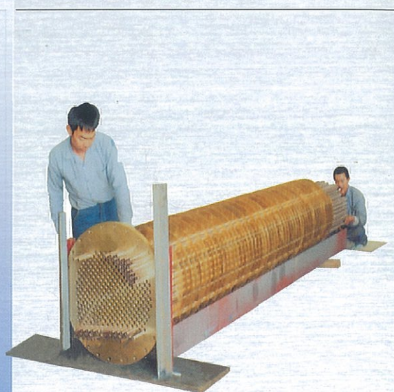
熱交換器製作中 Heat Exchanger
